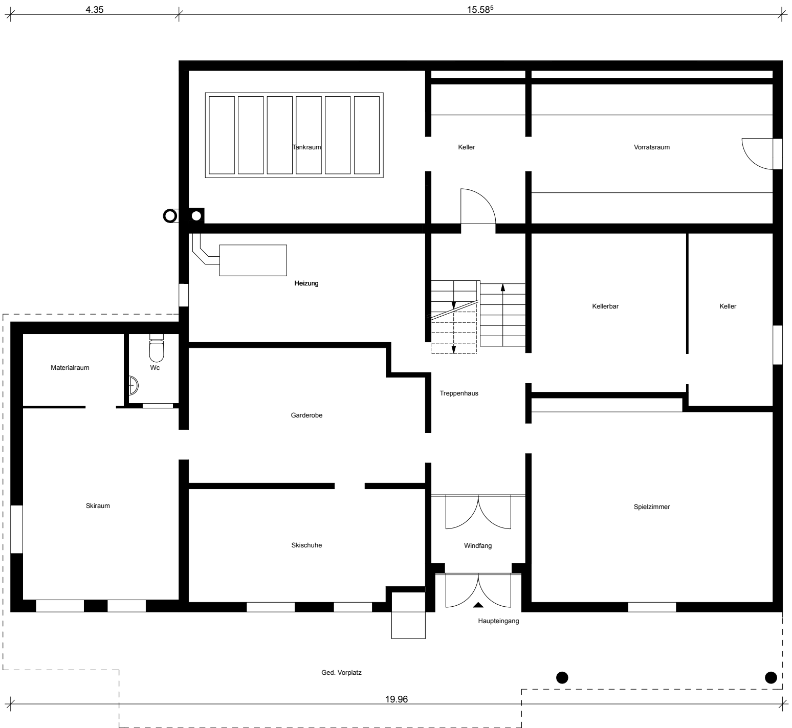
Skihaus Empächli, Untergeschoss Mst. 1 : 100
