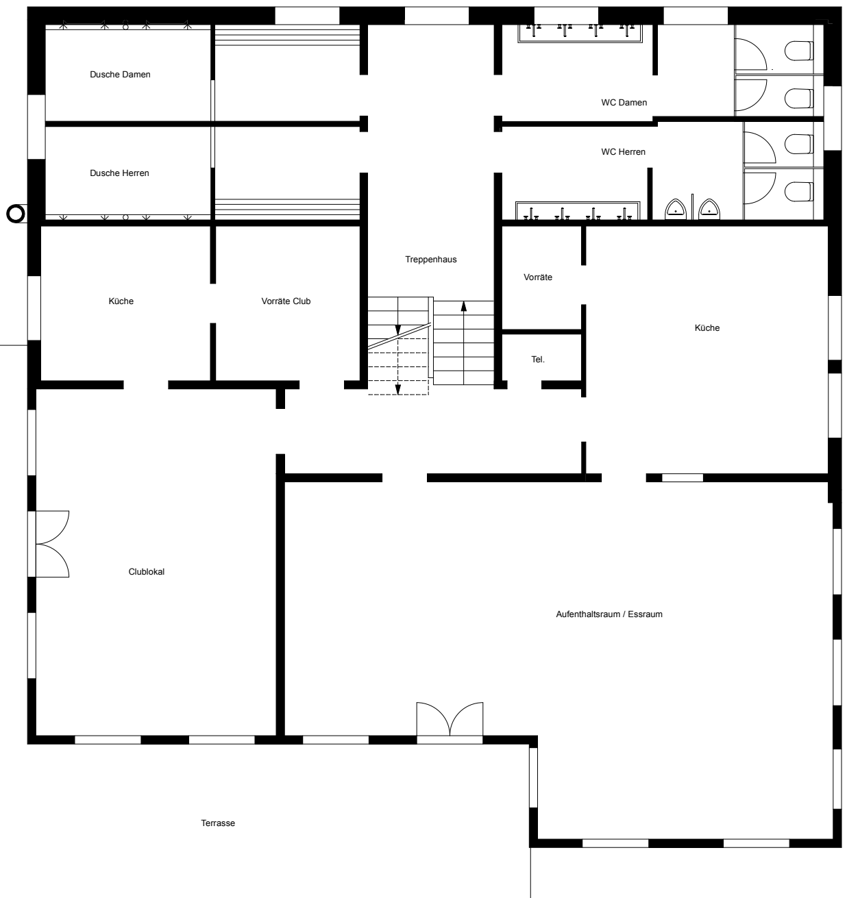
Skihaus Empächli, Erdgeschoss Mst. 1 : 100
